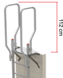
Altura de barandilla de 112 cm. Altura do gradil de 112 cm.
